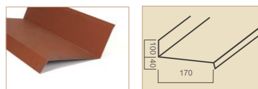
scossalina laterale aperta / open side flashing per rivestire il bordo laterale del pannello adiacente al muro. to cover the side edge of the panel adjacent to a wall.
