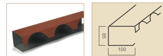
scossalina di testa / head flashing per rivestire il bordo superiore del pannello sporgente. to cover the upper edge of the protruding panel.
