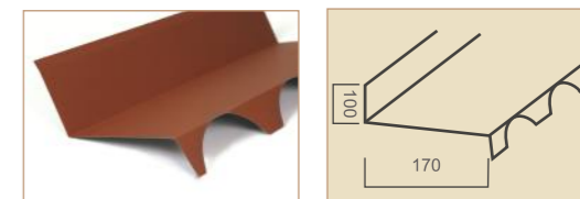
scossalina frontale con scanalature / front flashing with grooves per rivestire il bordo superiore del pannello adiacente al muro. to cover the upper edge of the panel adjacent to a wall.
