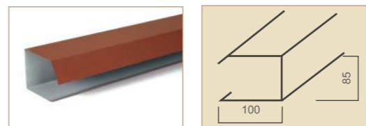
scossalina laterale chiusa / closed side flashing per rivestire il bordo laterale del pannello sporgente. to cover the side edge of the protruding panel.
